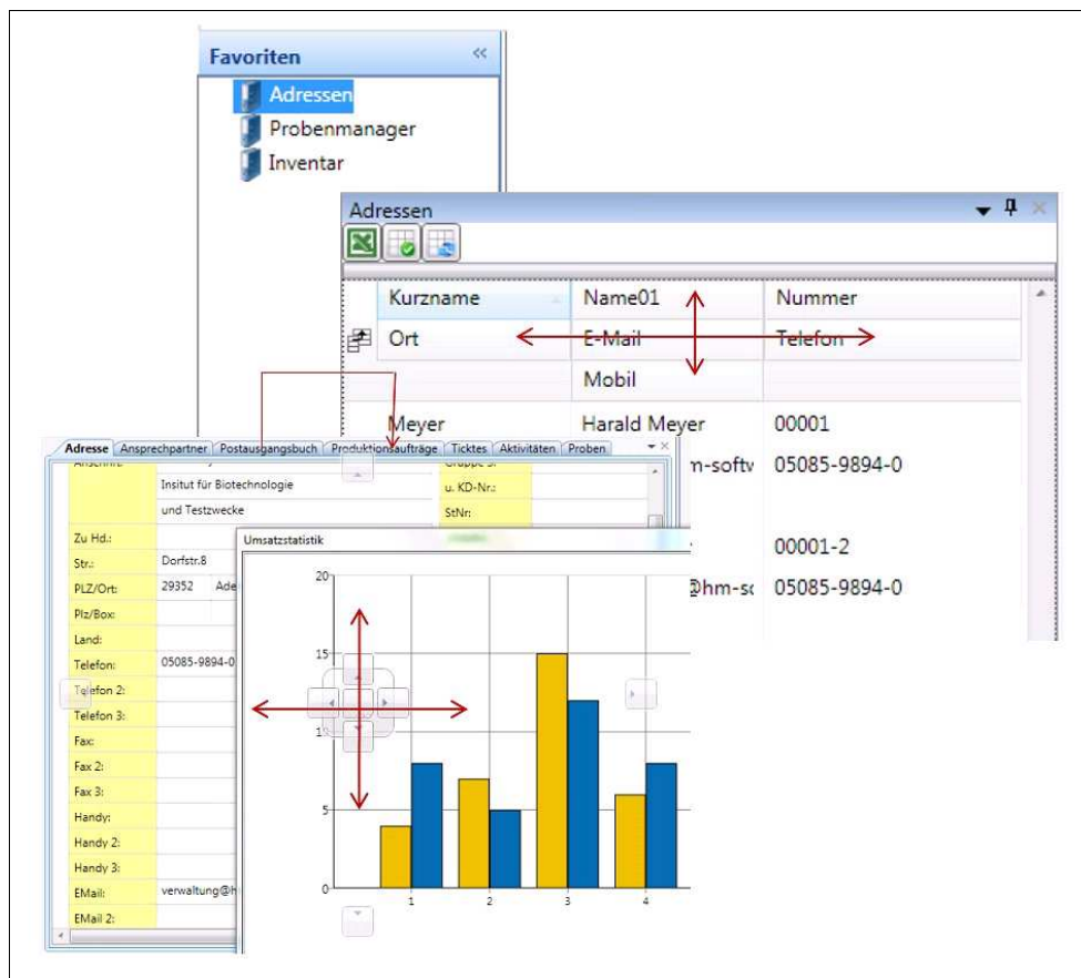
HM-LIMS 5.0: Neue flexible Anwenderoberfläche
